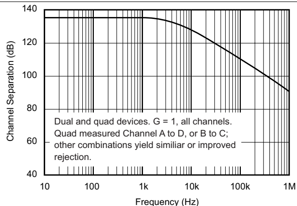
图 8. 通道分离与频率间的关系
