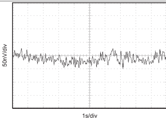
图 7. 输入噪声电压与时间的关系
