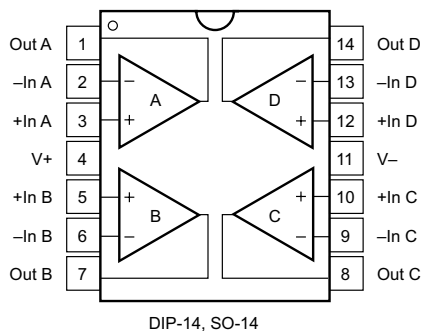
引脚功能: OPA227 和 OPA228
