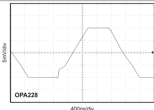
图 53. 大信号阶跃响应， G = 2 ， C_{LOAD} = 100pF ，输入信号 = 5Vp-p
