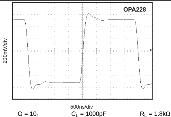
图 33. 小信号阶跃响应
