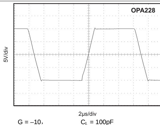
图 32. 大信号阶跃响应
