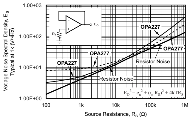
图 39. 采用单位增益缓冲器配置的 OPA227 的噪声性能
