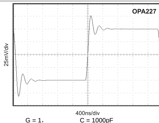
图 28. 小信号阶跃响应
