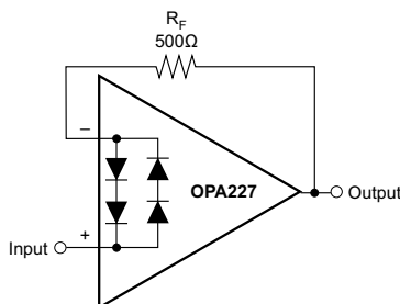
图 37. 脉冲操作
