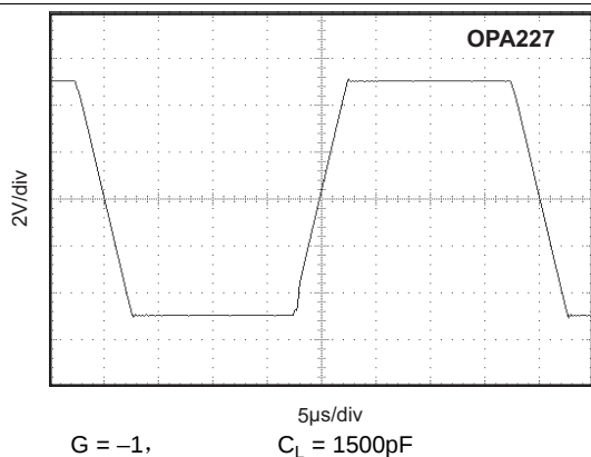
图 27. 大信号阶跃响应
