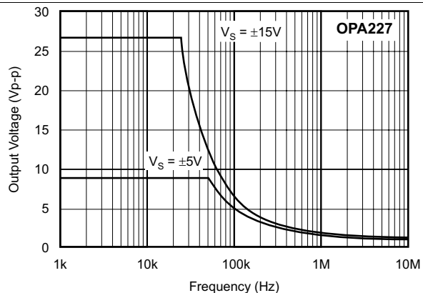
图 25. 最大输出电压与频率间的关系
