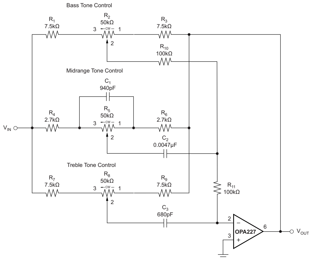
图 49. 三频主动音调控制（低音、中音和高音）
