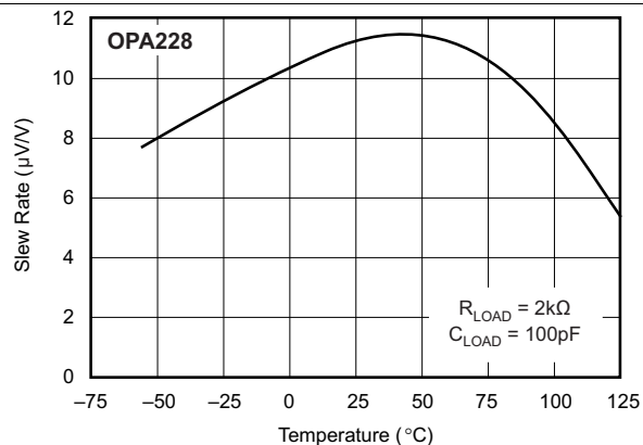
图 20. 压摆率与温度间的关系
