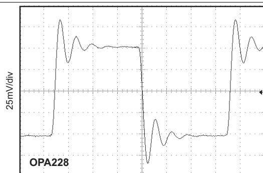
图 55. 小信号阶跃响应, G = 2 , C_{LOAD} = 100\text{pF} , 输入信号 = 50mVp-p。
