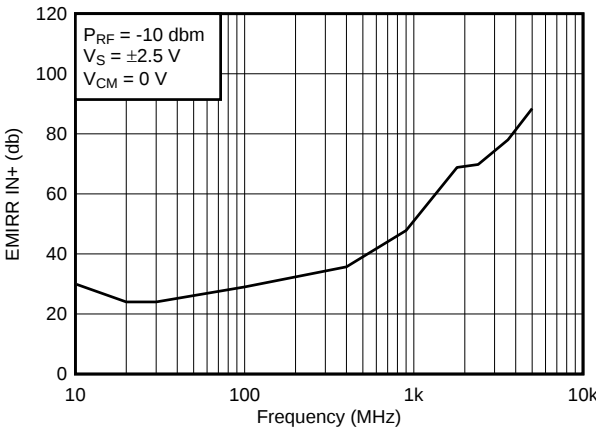
图 43. OPA227 EMIRR IN+ 与频率间的关系
